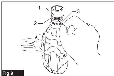
Fig. 9 ► 1. Impact socket 2. O-ring 3. Pin
