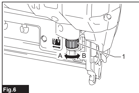
Fig.6 ► 1. Depth adjuster
