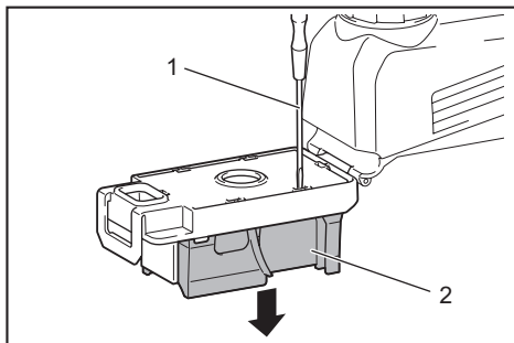
► 1. Destornillador de punta plana 2. Caja del filtro
