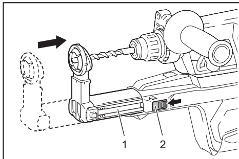
► 1. Guide 2. Guide adjustment button
